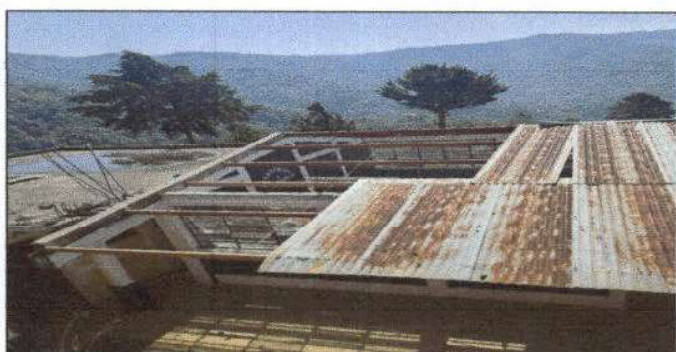
Foto 5: Sustitución de láminas troquelada aluzinc calibre 26
